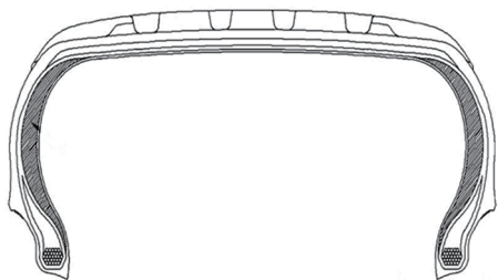
图3 RFT技术的结构示意图
